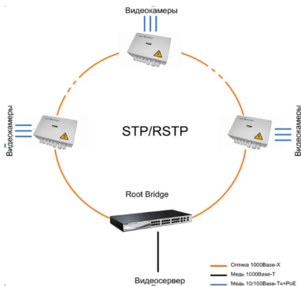
Рис. 2.2.17.1 Топология типа «кольцо»
