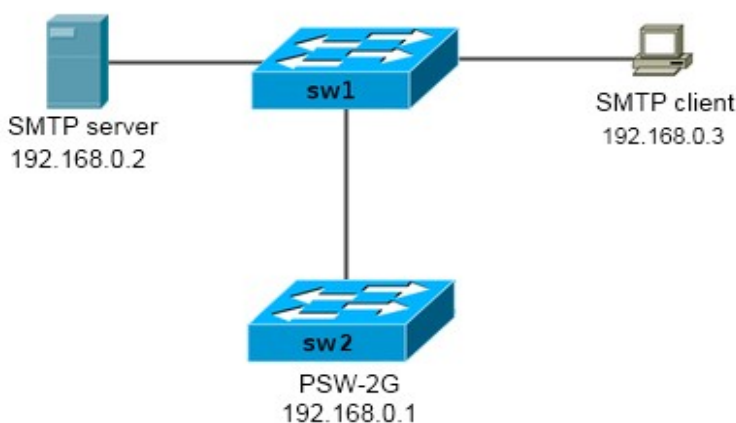
Рис. 2.2.12.1.1 Структура сети
