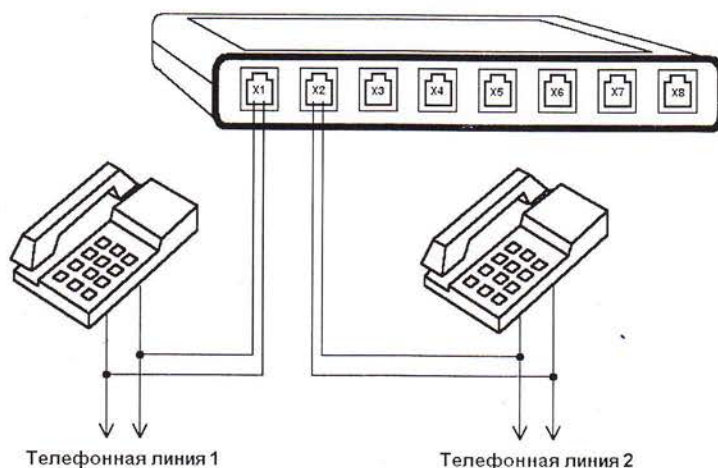
Схема 1. Подключение адаптера к телефонной сети общего пользования
