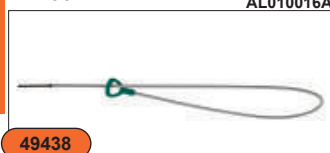
Щуп контроля уровня жидко- сти GMT MB 722.7**, 722.5**, оригинальный № 168 589 01 21 00 AL010016A
