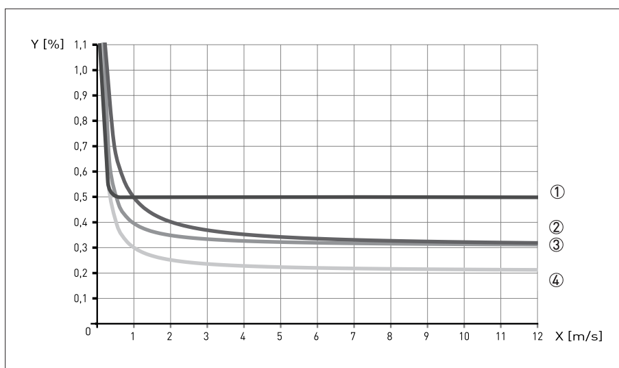
Рисунок 2-3: Зависимость погрешности от скорости потока
