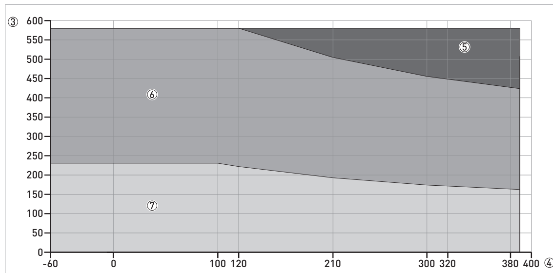
Рисунок 2-6: Номинальное давление / температура (ASME B16.5), фланцевое и резьбовое присоединение, в \text{°F} и фунт/кв.дюйм изб
