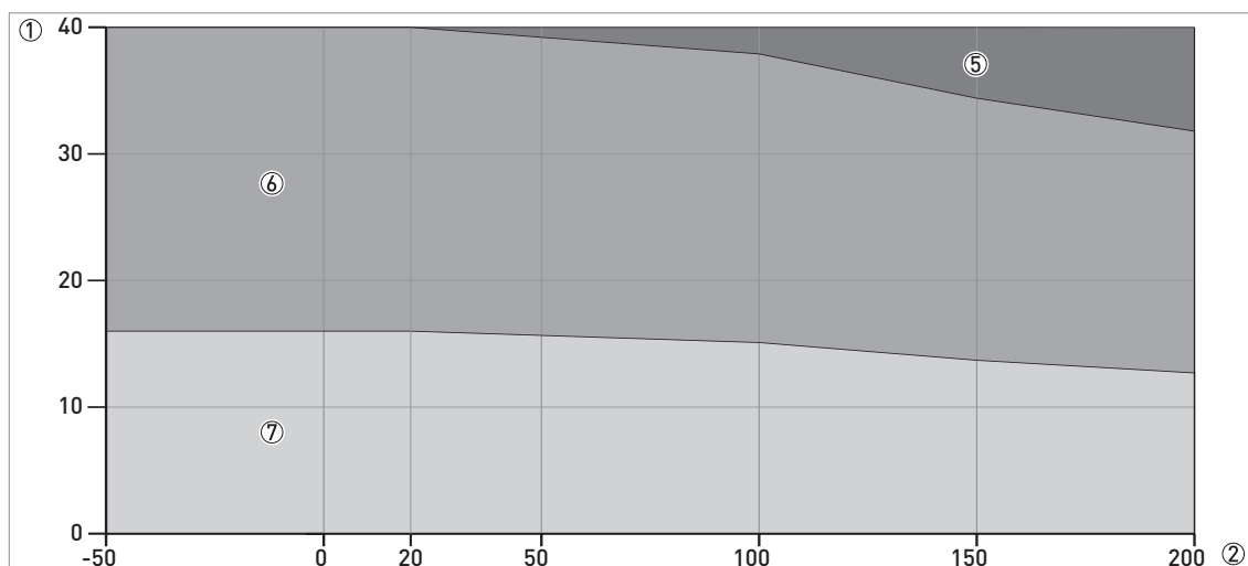
Рисунок 2-3: Номинальное давление / температура (EN 1092-1), фланцевое и резьбовое технологическое присоединение, в \bar{A} и \bar{B} бар изб
