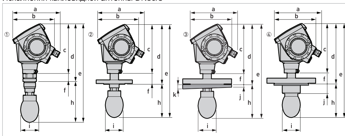
Рисунок 2-12: Исполнения каплевидной антенны DN80/3"
