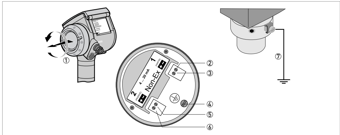
Рисунок 4-1: Электрическое подключение
