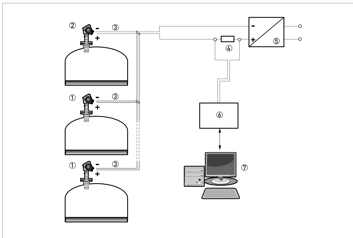
Рисунок 4-5: Сеть с многоточечным подключением (для приборов невзрывозащищенного исполнения)
