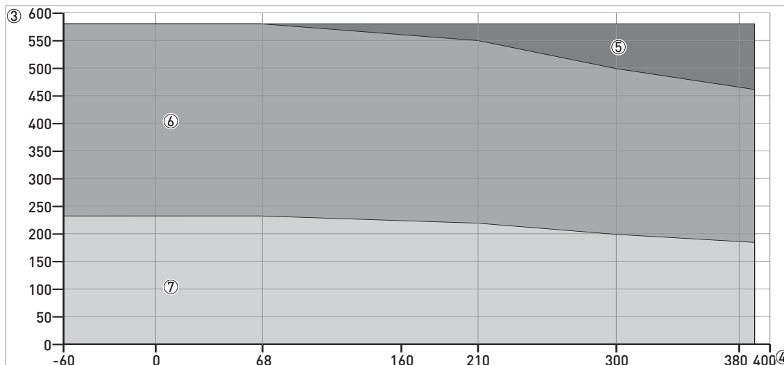
Рисунок 2-4: Номинальное давление / температура (EN 1092-1), фланцевое и резьбовое технологическое присоединение, в \bar{A} и \bar{B} фунт/кв.дюйм изб
