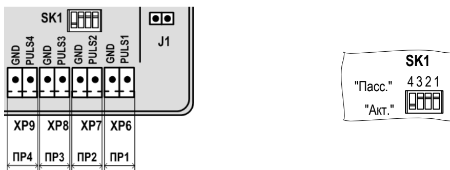
Рис.10. Маркировка коммутационных элементов подключения ПР.
