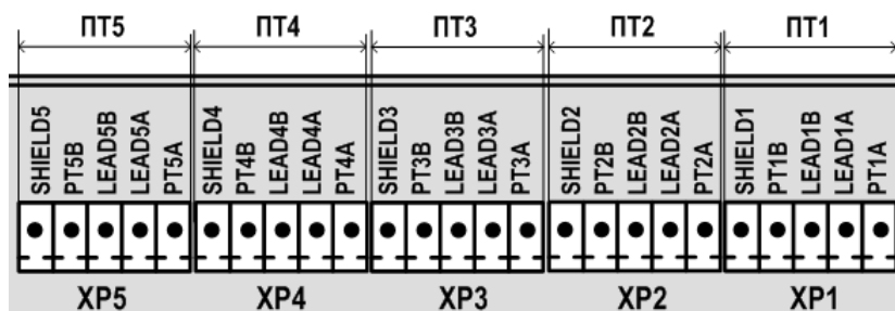
Рис.12. Обозначение коммутационных элементов подключения ПТ.
