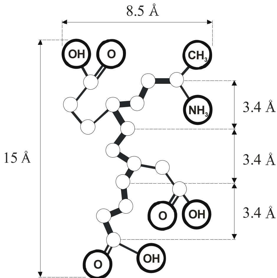
Рис. 13. Развернутая конформация пептида Ala-Glu-Asp-Gly (проекция на плоскость). Представлены концевые и боковые функциональные группы, способные к комплементарным взаимодействиям с ДНК.
