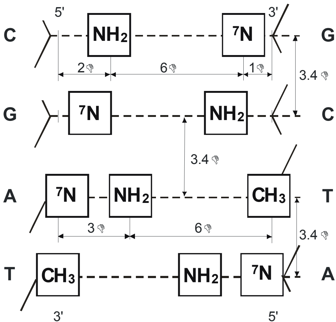
Рис. 14. Метрическое расположение функциональных групп на поверхности большой канавки при встраивании каждой нуклеотидной пары в двойную спираль ДНК.
