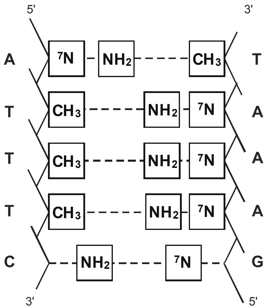
Рис. 15. Последовательность нуклеотидных пар в двойной спирали ДНК, функциональные группы которой комплементарны функциональным группам пептида Ala-Glu-Asp-Gly .
