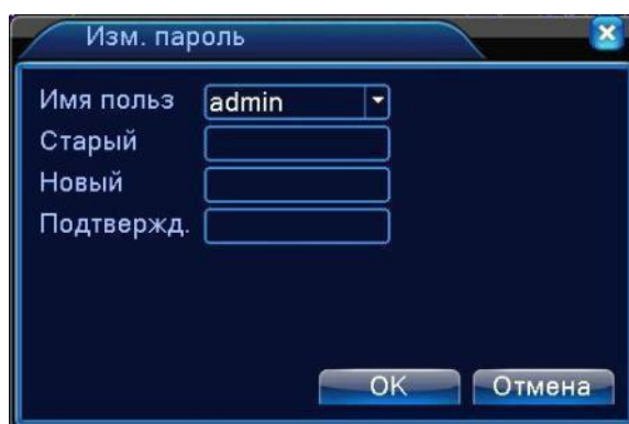
Рисунок 4.36 Изменить пароль
