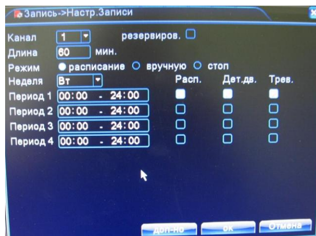
Рисунок 4.1 Настройка записи
