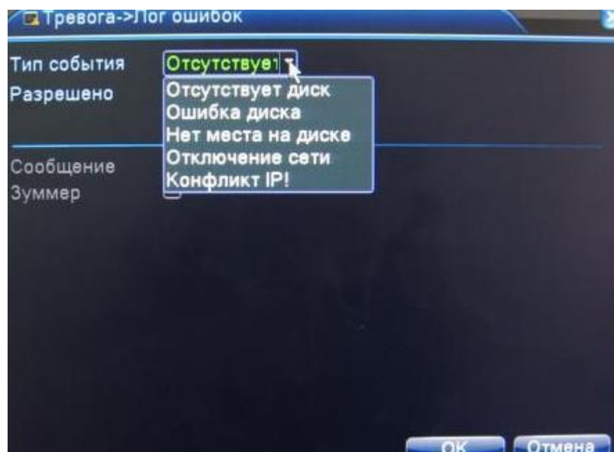
Рисунок 4.8 Лог ошибок
