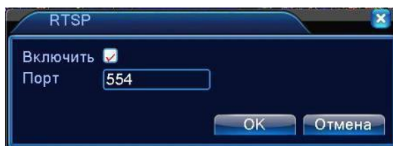
Рисунок 4.27 Настройка RTSP
