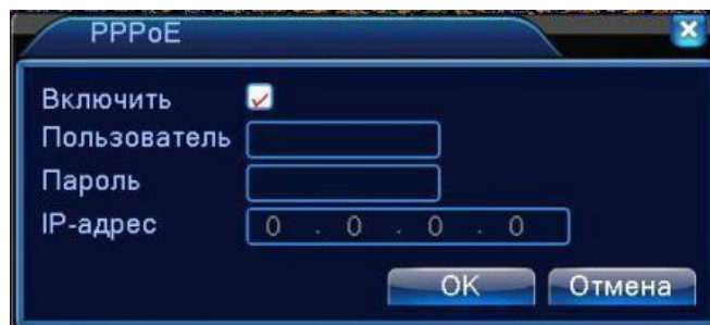
Рисунок 4.15 PPPoE
