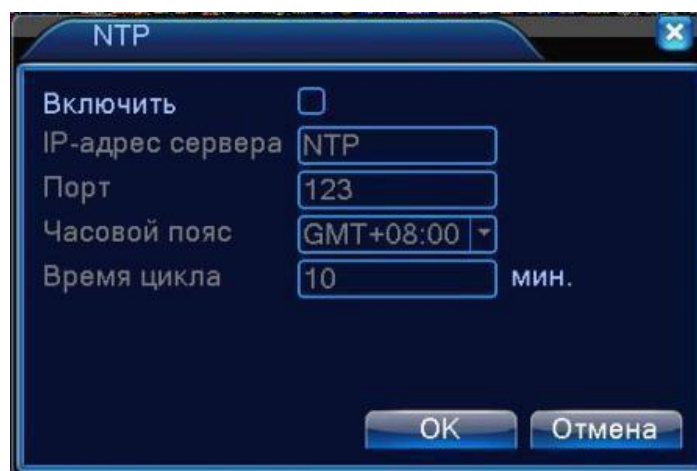
Рисунок 4.16 NTP
