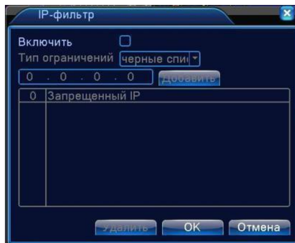
Рисунок 4.18 IP-фильтр
