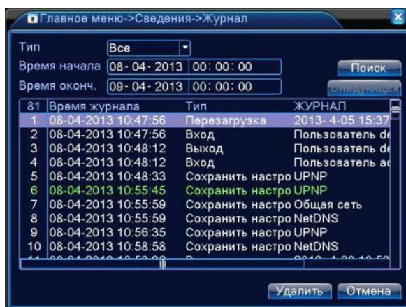
Рисунок 4.48 Информация журнала
