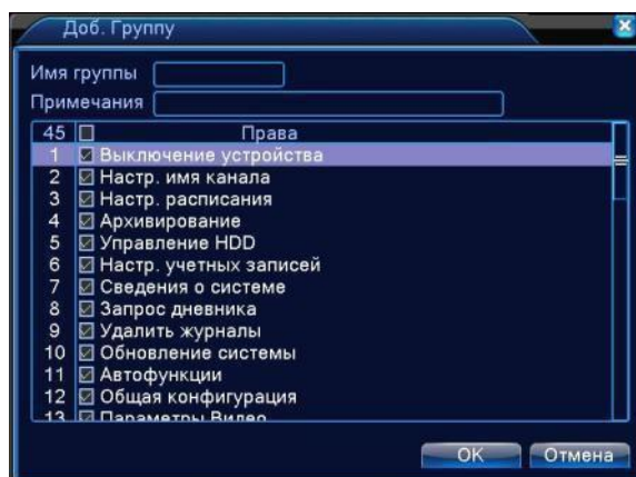
Рисунок 4.38 Добавить группу
