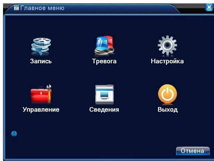
Рисунок 3.3 Главное меню
