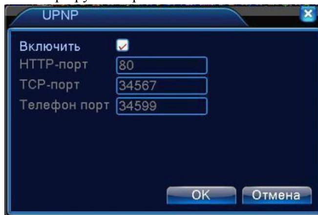
Рисунок 4.25 UPNP
