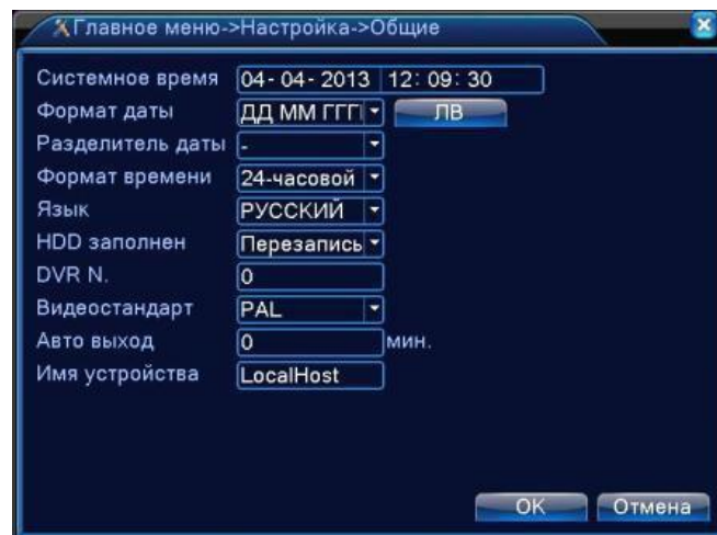
Рисунок 4.9 Общие настройки
