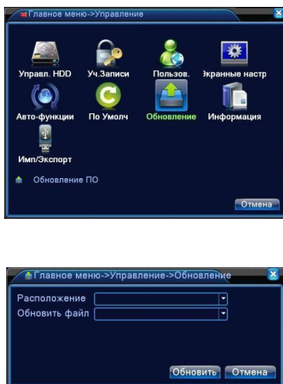
Рисунок 4.43 Обновление
