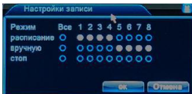
Рисунок 3.6 Режимы записи
