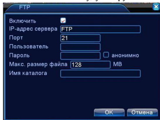
Рисунок 4.20 Настройки FTP
