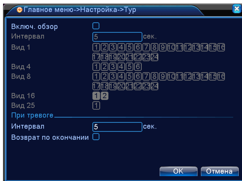
Рисунок 4.29 Настройка переключения
