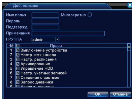
Рисунок 4.37 Добавление пользователя
