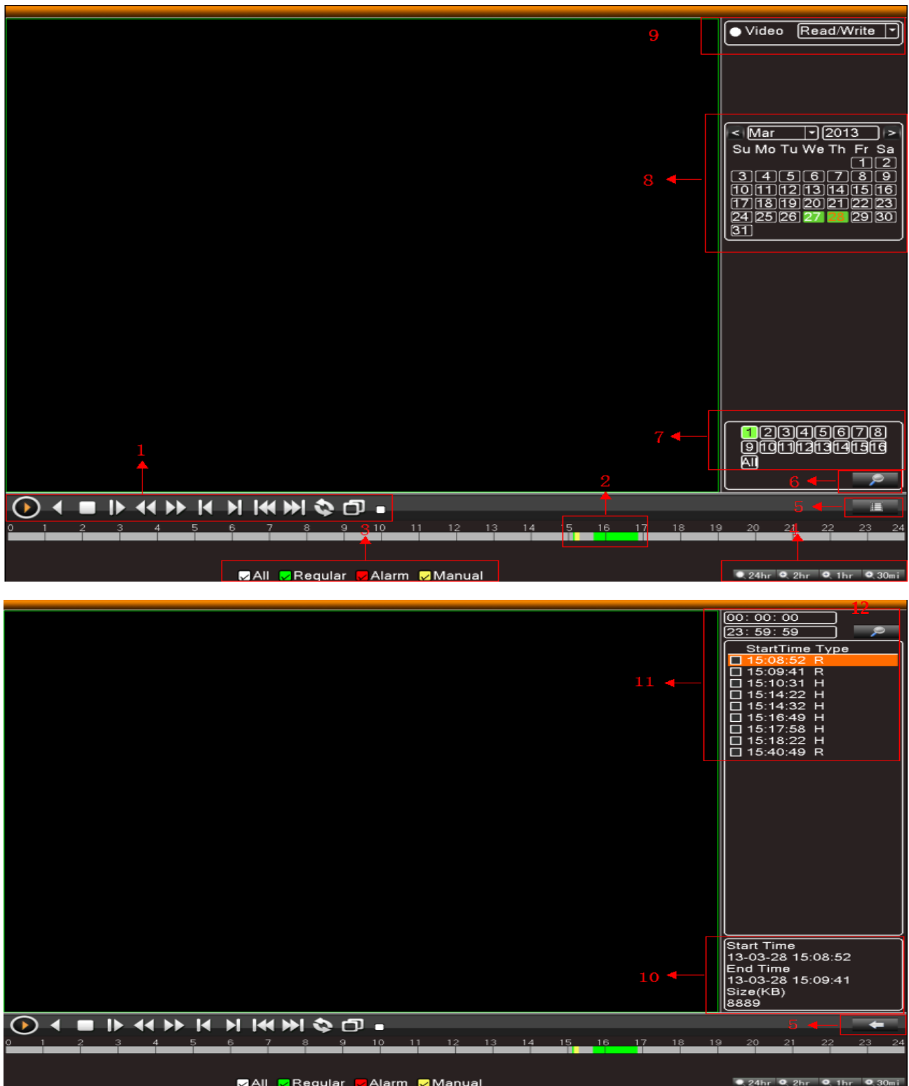
Рисунок 3.4 Воспроизведение видео
