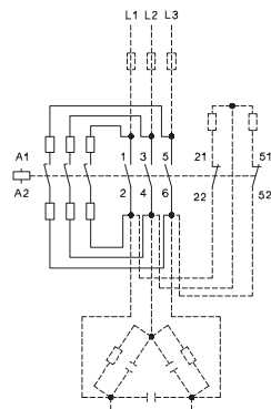
Принципиальная схема с быстроразрядными резисторами
