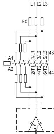
Стандартная принципиальная схема Типоразмеры 0 и 3
