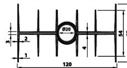
Сечение секции
