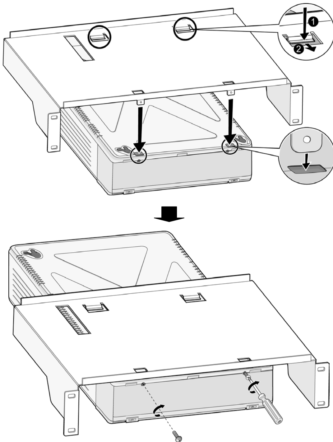
Рис. 3.2.7.2б Установка стоечного крепления
