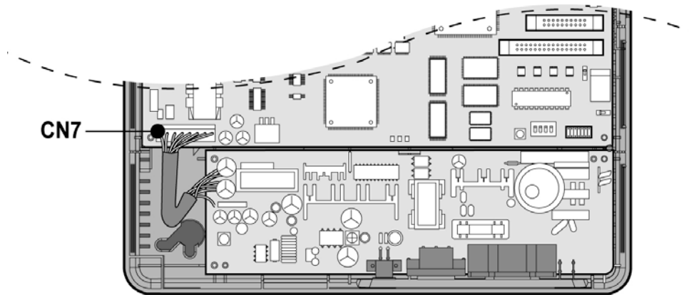
Рис. 3.2.4а Установка блока питания
