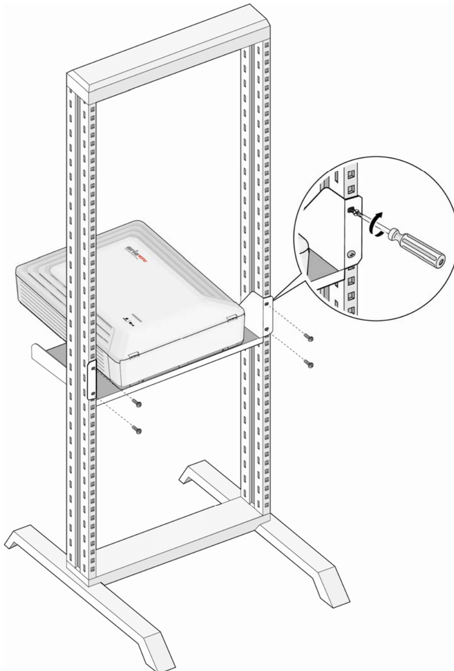
Рис. 3.2.7.2а Монтаж системного блока в стойке
