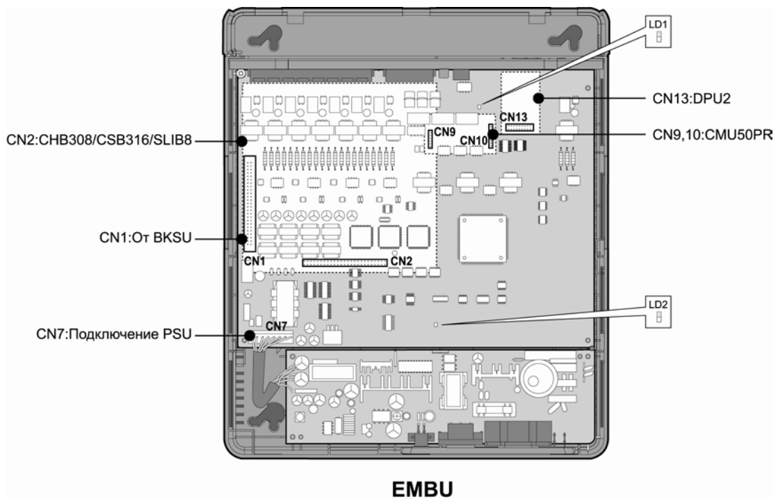
Рис. 4.3а Материнская плата блока расширения (EMBU)
