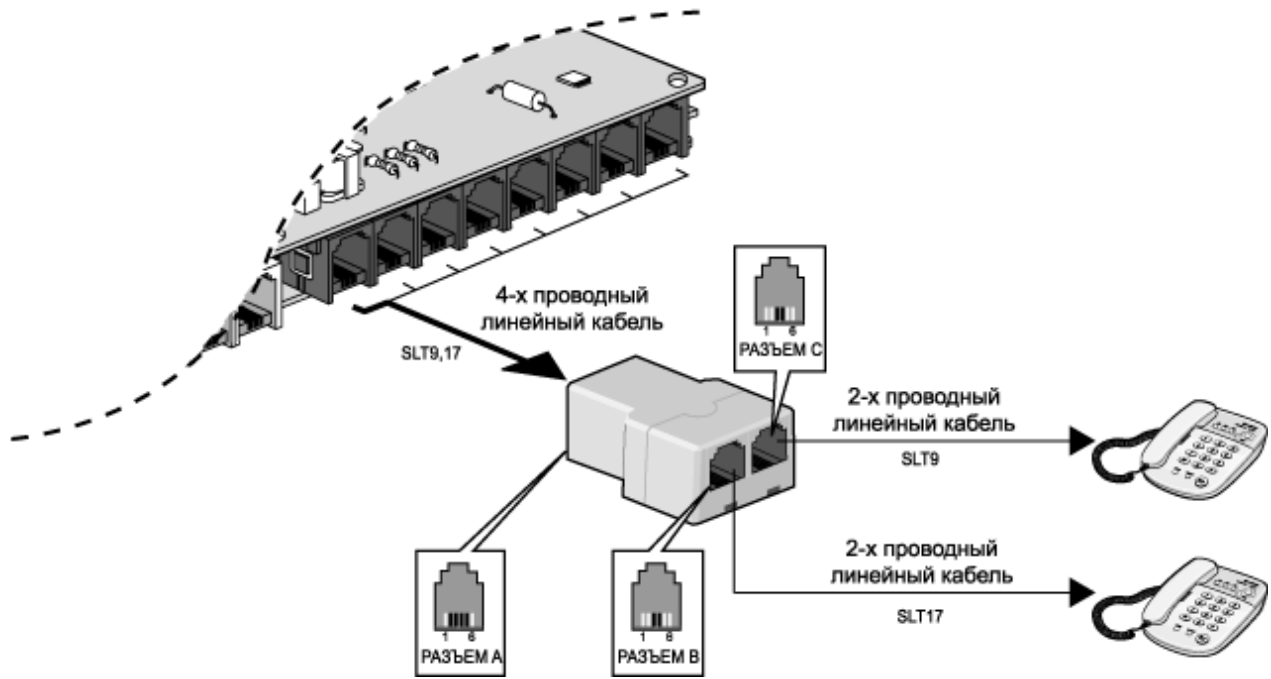
Рис. 4.4.2.2 Терминальный переходник
