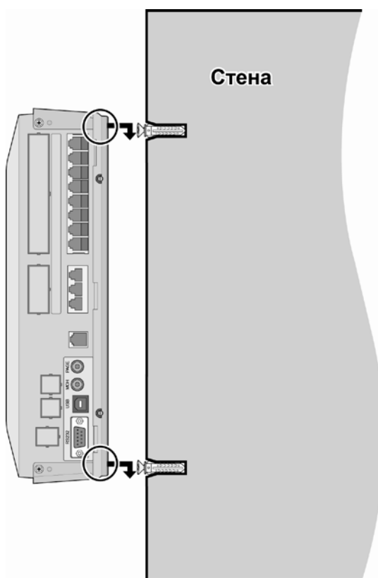
Рис. 3.2.7.16 Настенный монтаж системного блока
