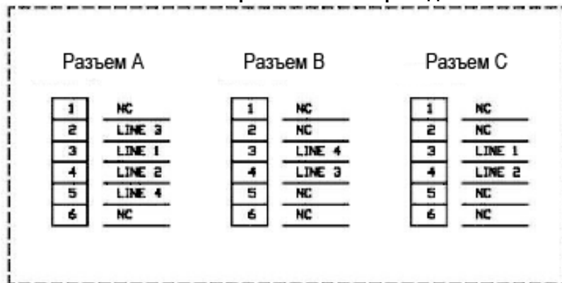
Рис. 4.4.2.2 Терминальный переходник
