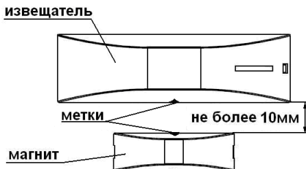
Рис. 11 Общий вид извещателя Репид-Р2
