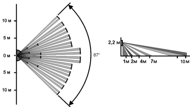
Рис.8 Диаграмма зоны обнаружения
