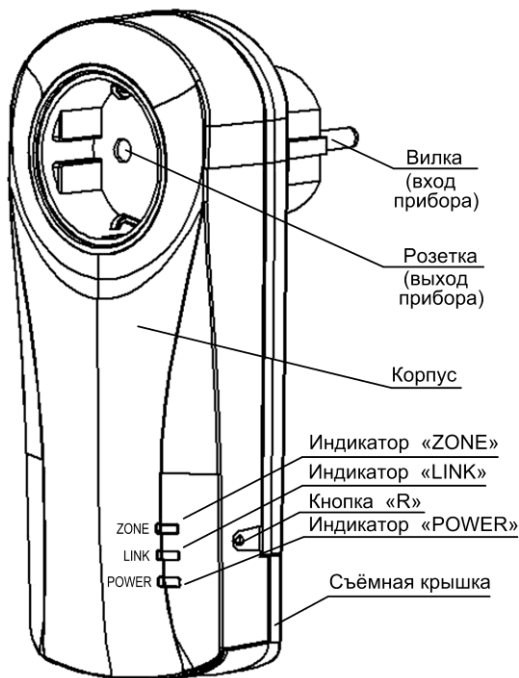
Рис.1 Внешний вид GSM розетки
