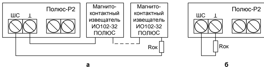
Рис. 12 Схема подключения извещателя
